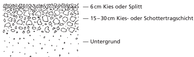
Kies-Splitt-Decke
